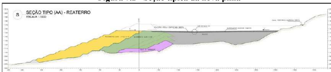
Figura 7.2 - Seção típica da nova pilha
