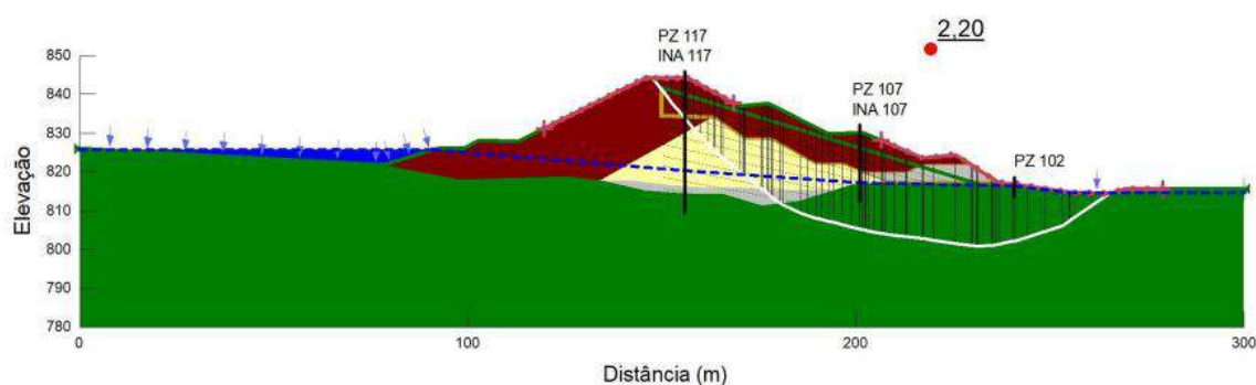
Figura 6 - Linha freática obtida para condição atual da Barragem B1.
