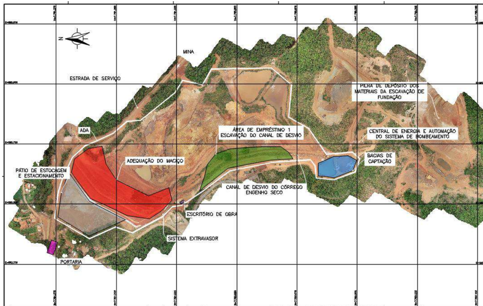
Figura 1 - Arranja Geral das Obras
