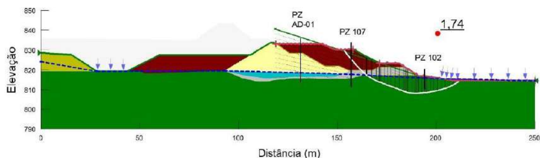
Figura 9 – Análise de estabilidade considerando carregamento dinâmico da seção crítica D-D' da Barragem B1.
