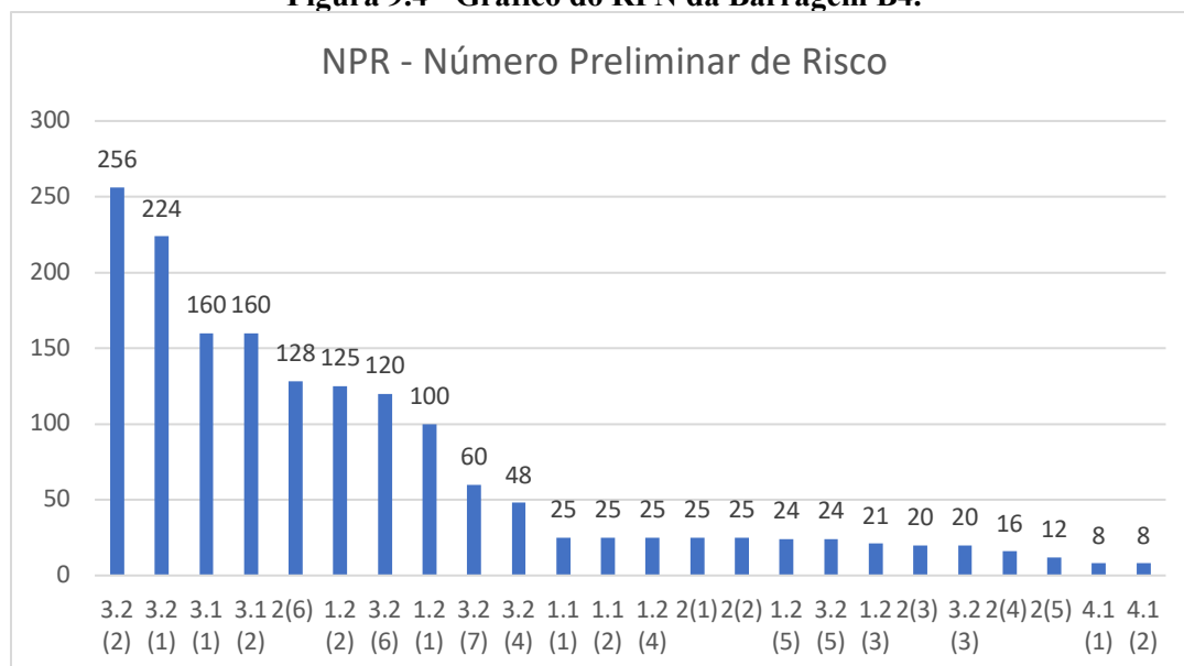
Figura 9.4 - Gráfico do RPN da Barragem B4.
