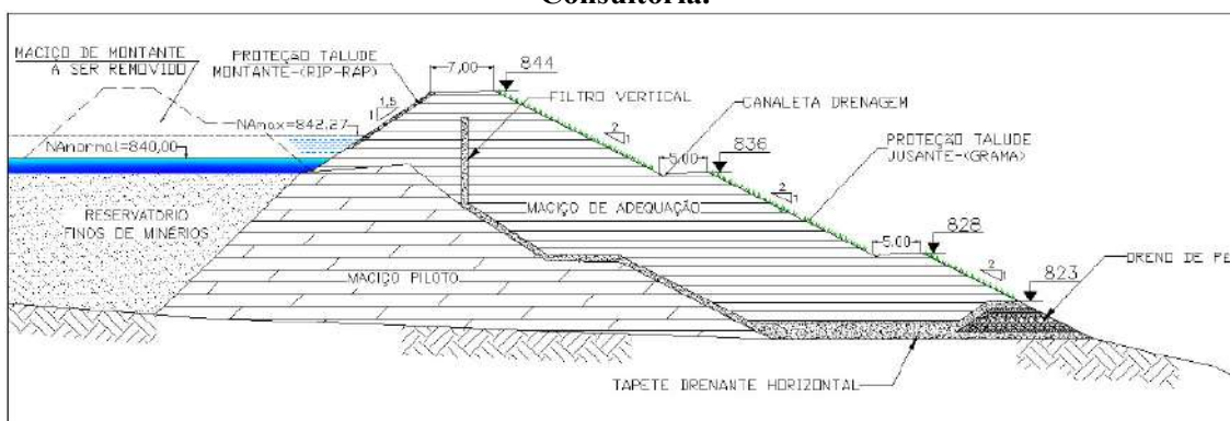
Figura 7.1 - Seção Típica de adequação - Fonte: projeto da GEO GRAPHOS Engenharia e Consultoria.
