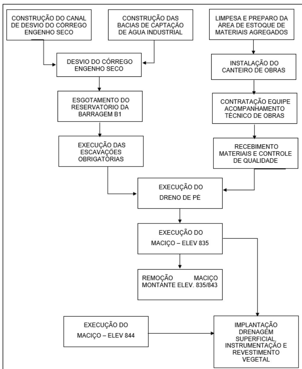
Figura 2 - Fluxograma das obras de descaracterização da Barragem B1
