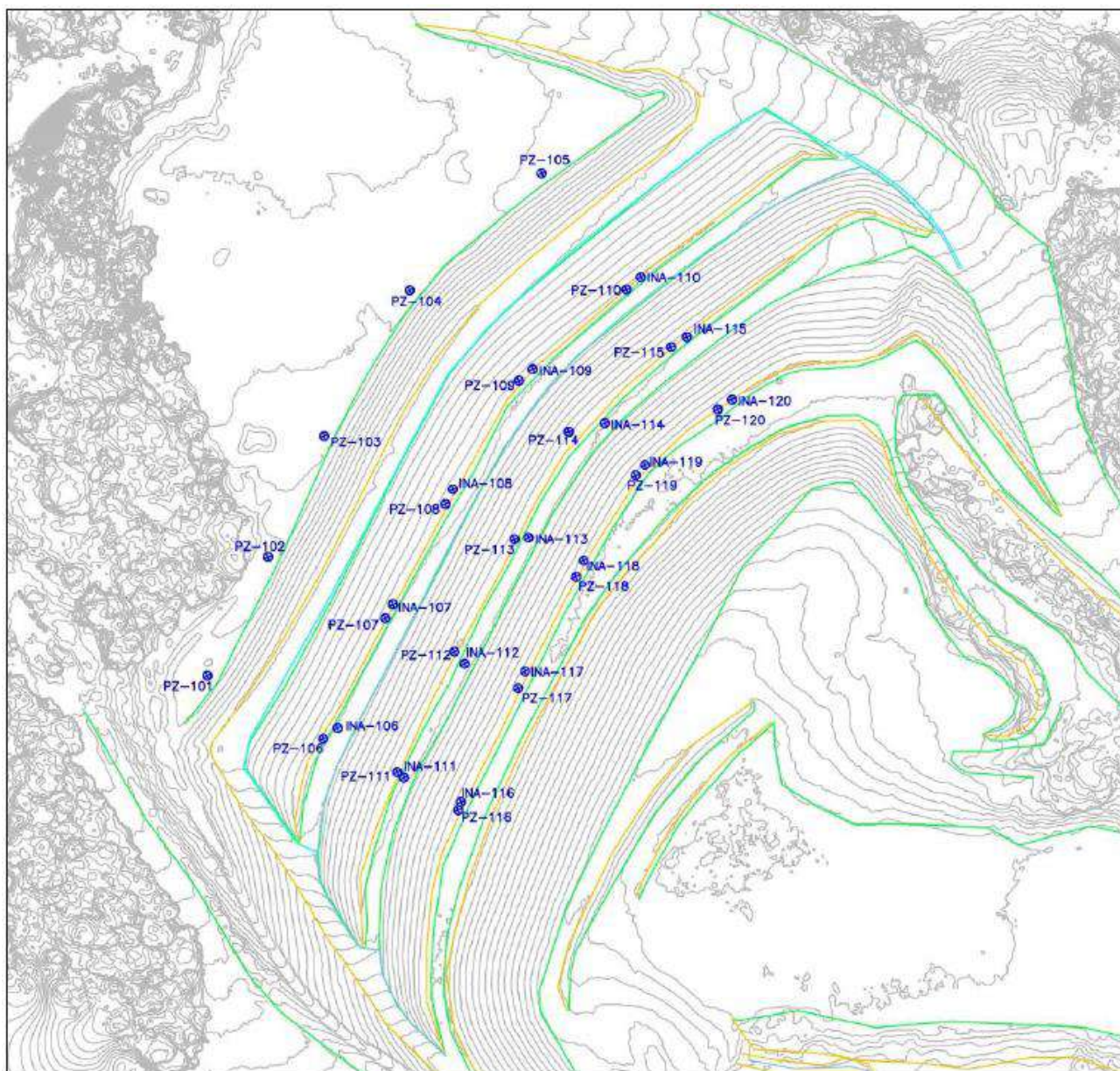
Figura 13 - Vista geral da instrumentação instalada na Barragem B1.
