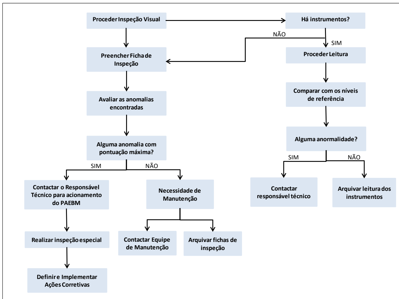
Figura 10 – Fluxograma de atividades de inspeção regular.
