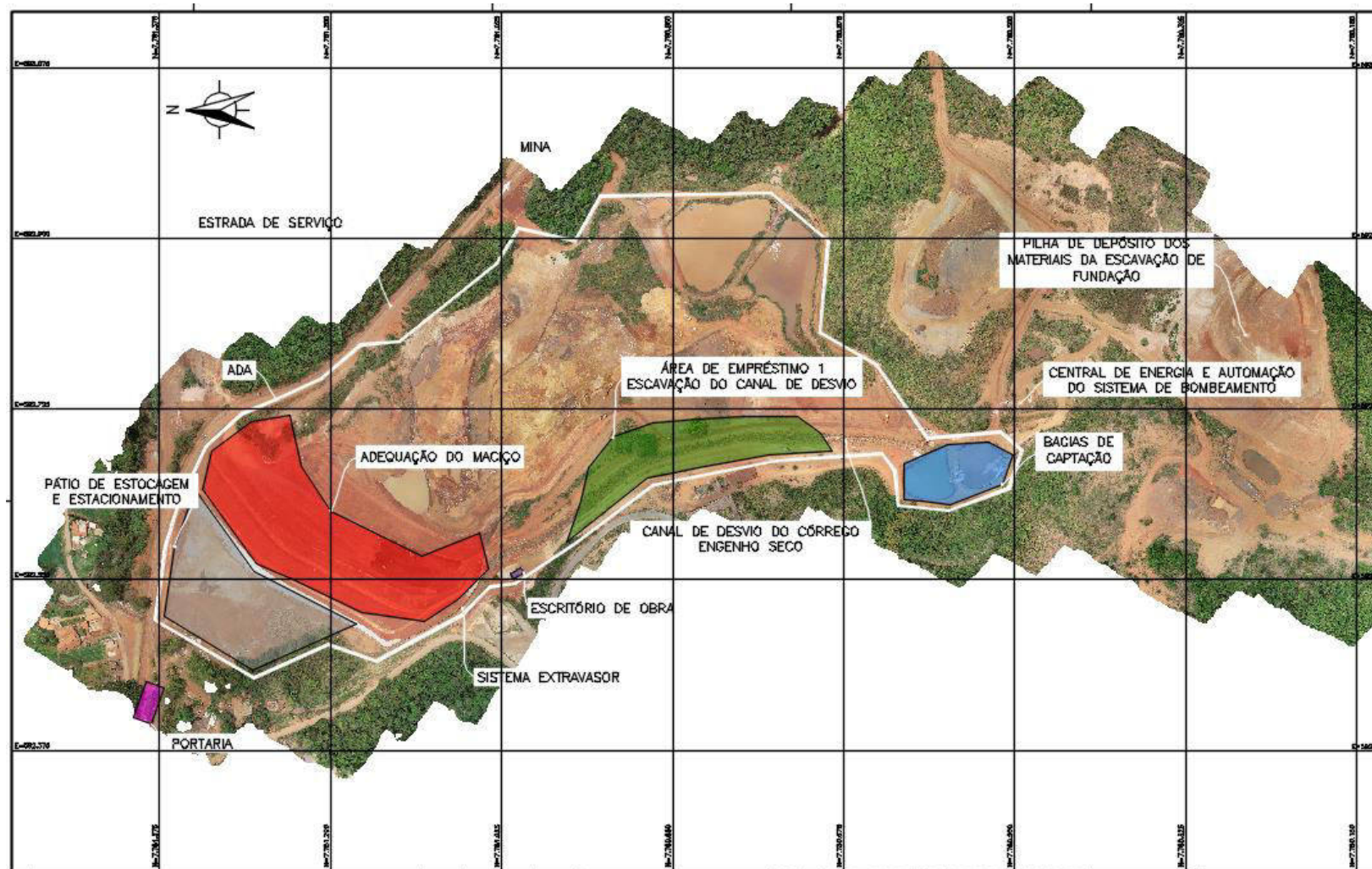
Figura 1 - Arranjo Geral das Obras
