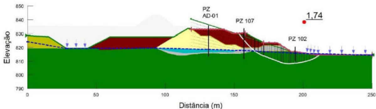
Figura 9 – Análise de estabilidade considerando carregamento dinâmico da seção crítica D-D' da Barragem B1.
