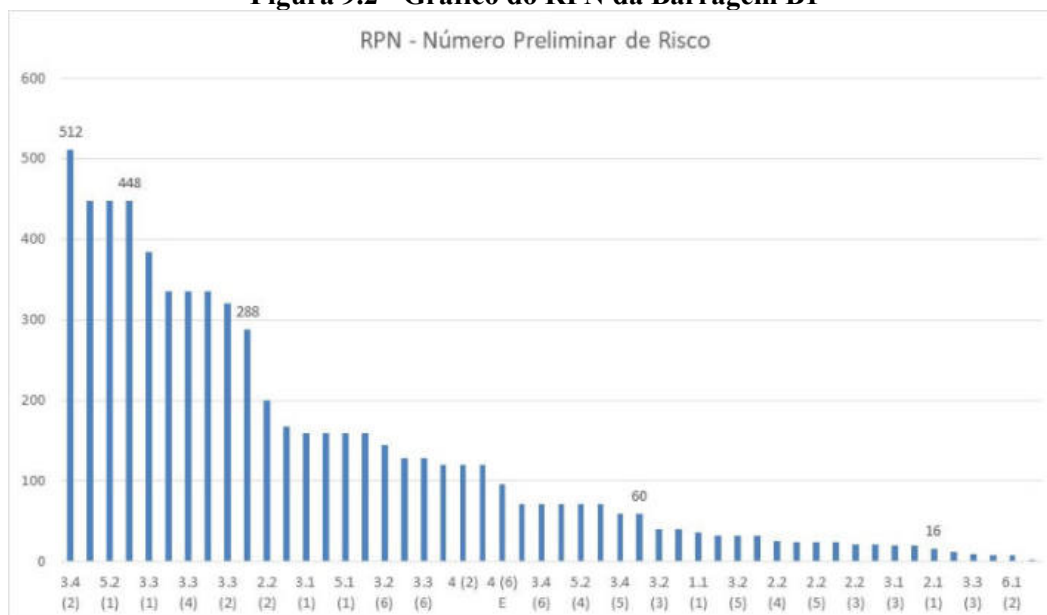
Figura 9.2 - Gráfico do RPN da Barragem B1
