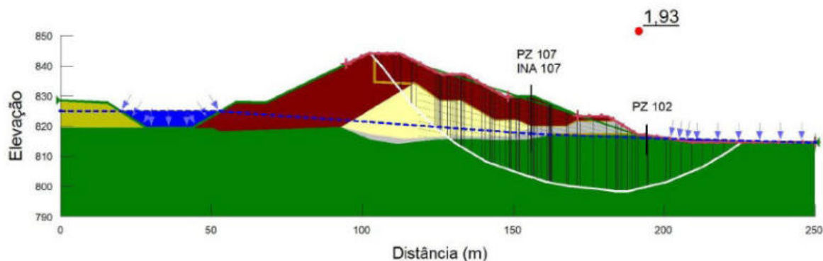
Figura 6 - Linha freática obtida para condição atual da Barragem B1.
